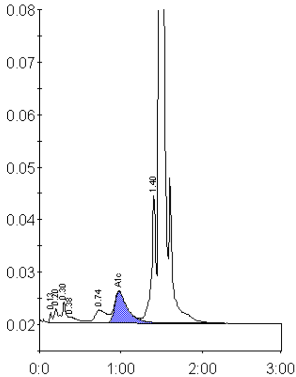
Peak table - ID: 10576158
